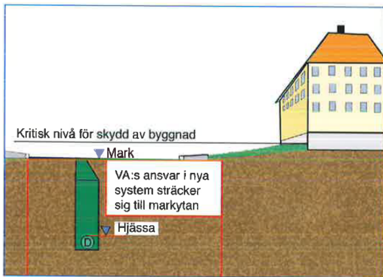
Figur 5. Dagvattenhanteringens tre dimensioneringsnivåer (Svenskt Vatten, 2019).
